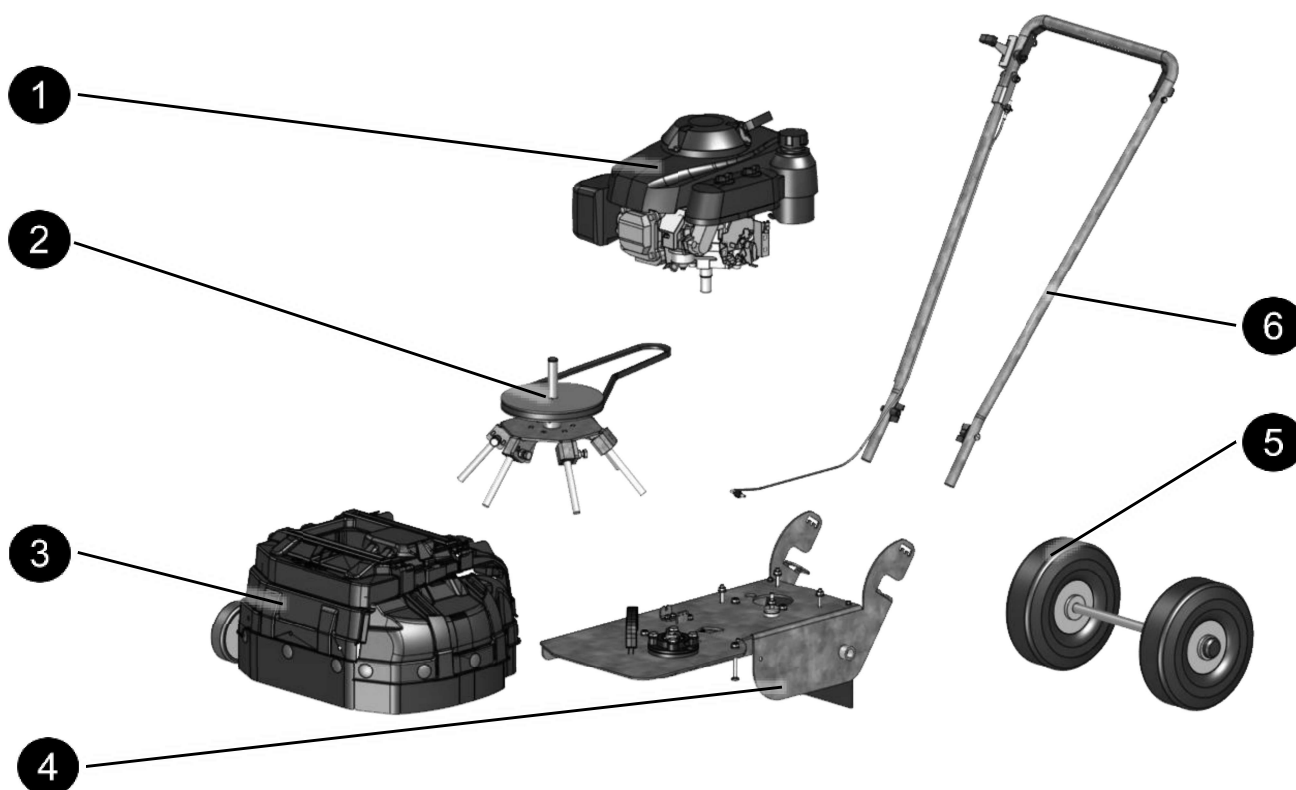
Abbildung 19: Ersatzteilübersicht
