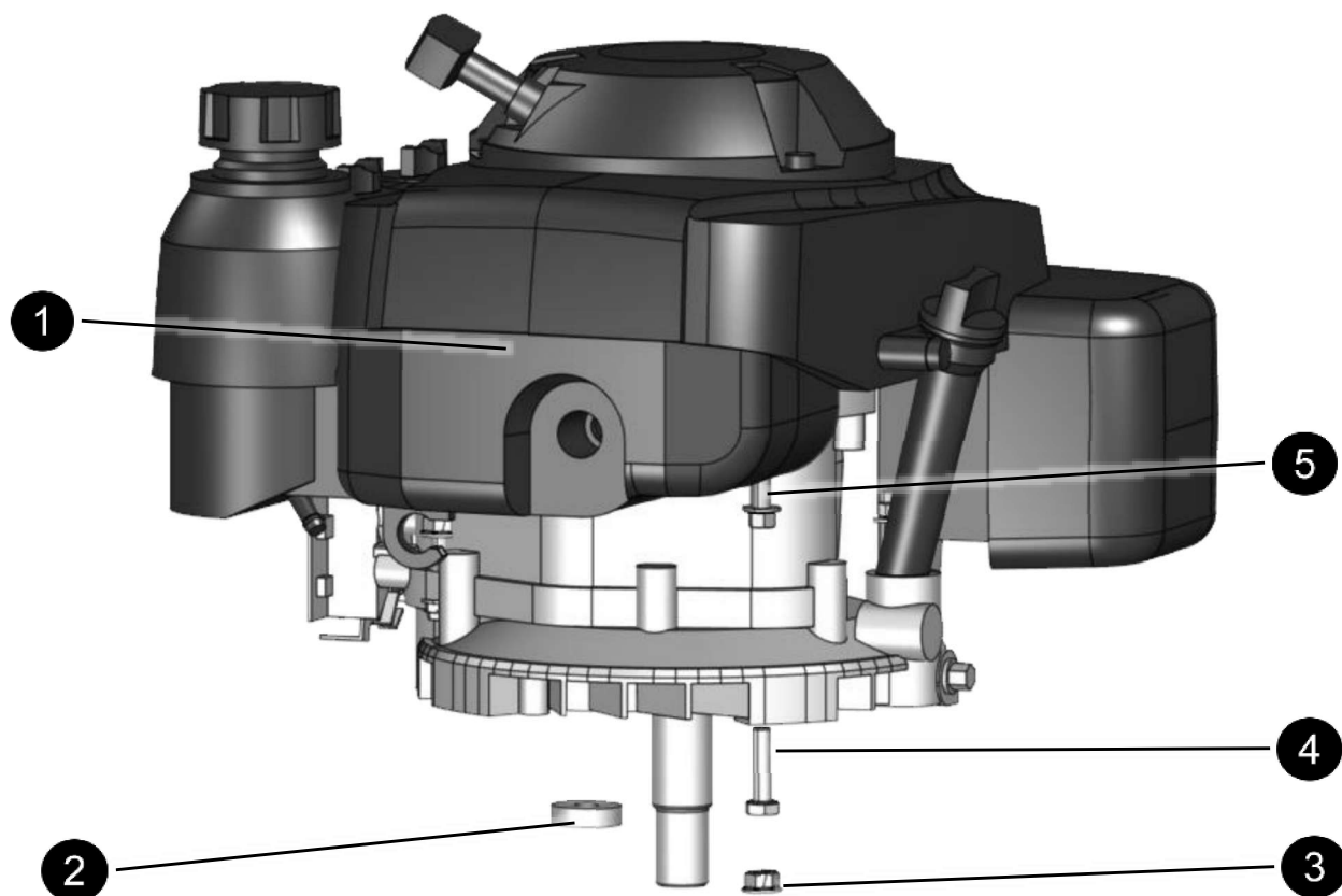
Abbildung 21: Motor Honda GXV 160 OHV Technik
