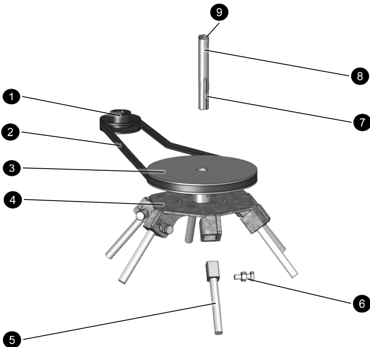
Abbildung 22: Antriebseinheit (1)
