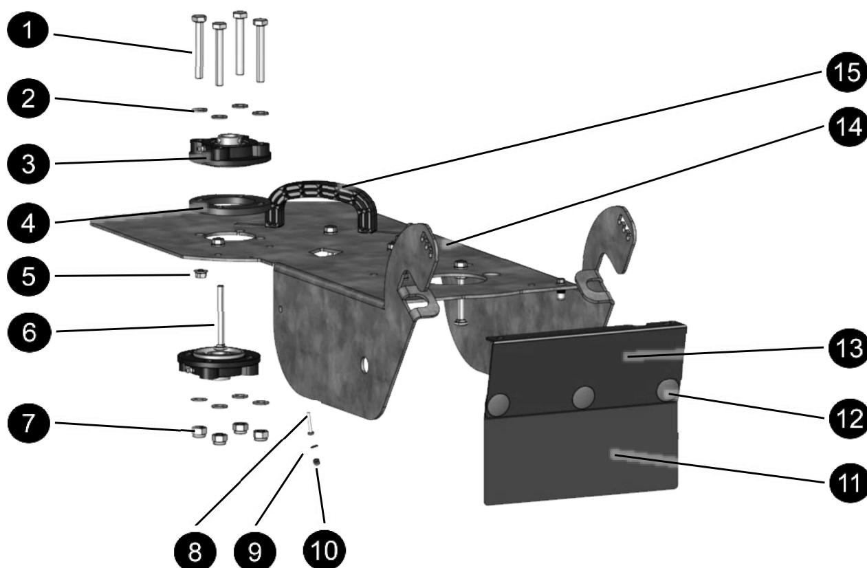
Abbildung 25: Grundrahmen
